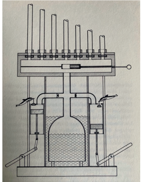
Hydraulos: Schema ©Hallwag
